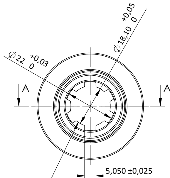
Tvar ze souboru SHAFT m1 20deg z31.dxf
