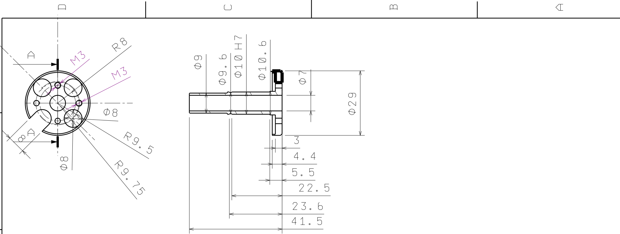
Front view Scale: 1:1
