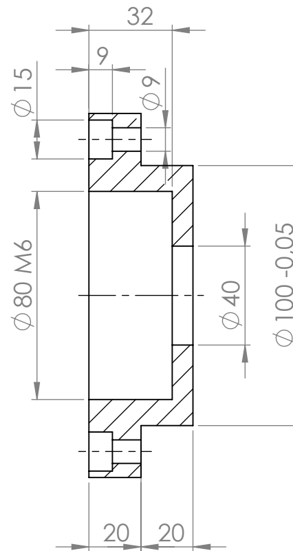
ŘEZ A-A
